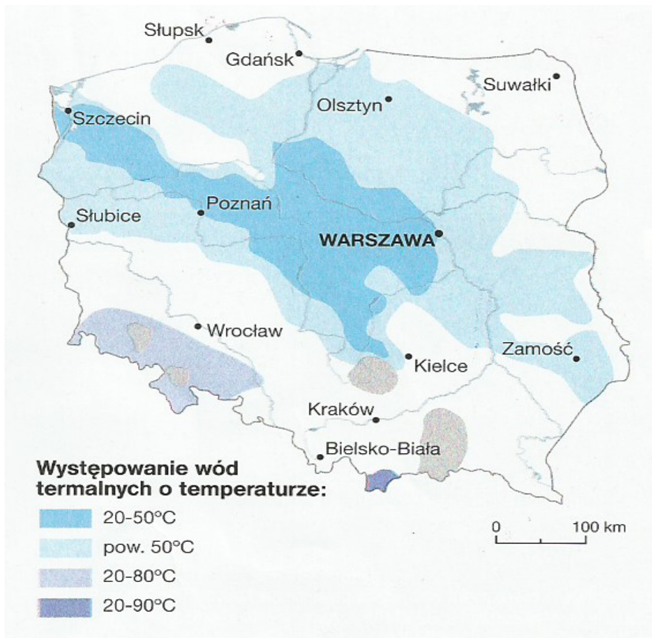
Rys.10. wody termalne; NATIONAL GEOGRAFIC –Listopad 2015 r.
