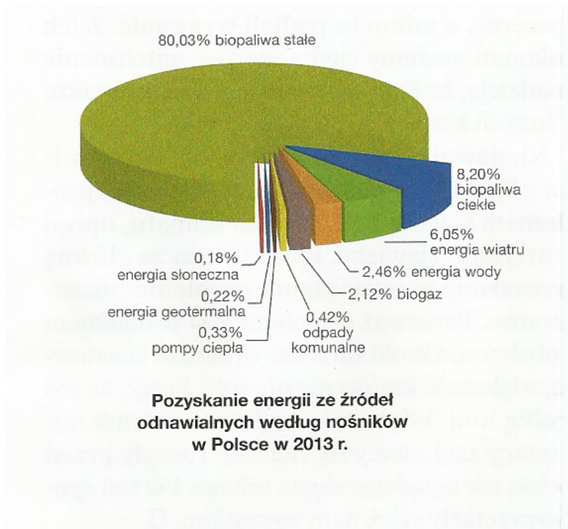
Rys.8. energia ze źródeł odnawialnych; NATIONAL GEOGRAPHIC –Listopad 2015 r.
